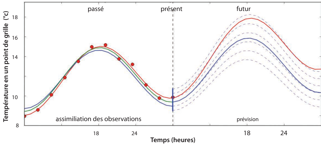
3 Illustration simplifiée de la mise en œuvre d'une assimilation de données variationnelle
