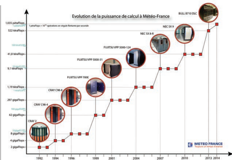
2 L'évolution de la puissance de calcul à Météo-France. L'unité flops correspond à une opération en virgule flottante par seconde ; 1 péta (P) = 10^{15} , 1 téra (T) = 10^{12} , 1 giga (G) = 10^9
