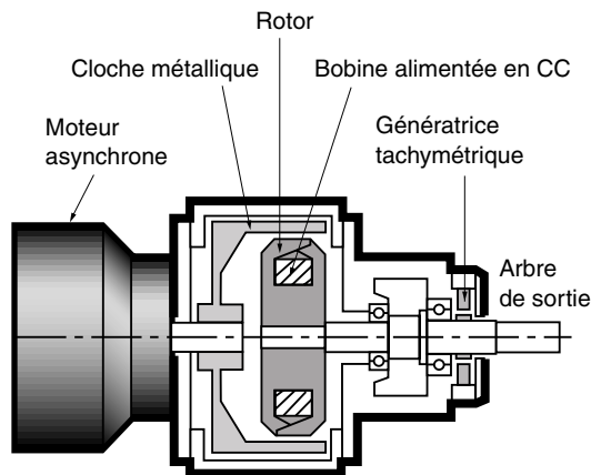
Fig. 20 : Coupe schématique d'un variateur de vitesse à courant de Foucault.
