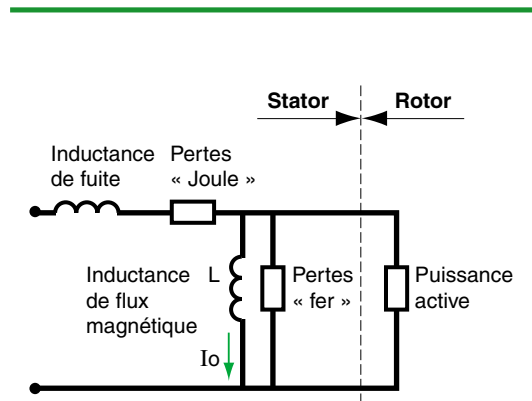
Fig. 17 : Schéma équivalent d'un moteur asynchrone.
