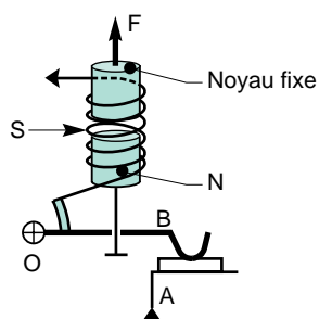
Fig. 7 : schémas de propulseurs de contacts électrodynamique à propre courant.
