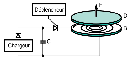
Fig. 5 : schéma d'un propulseur de contacts selon le principe de Elihu Thomson.
