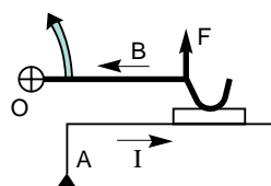
Fig. 6 : schémas de propulseurs de contacts à propre courant électrodynamique.
