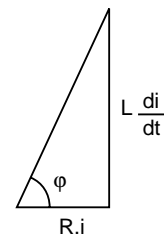
Fig. 3 : représentation vectorielle des deux composantes R i et L \frac{di}{dt} .
