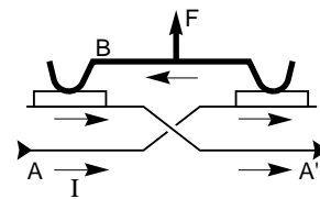
Fig. 6 : schémas de propulseurs de contacts à propre courant électrodynamique.
