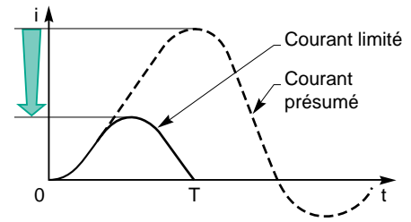
Fig. 1 : représentation des courants de court-circuit, présumé et limité.
