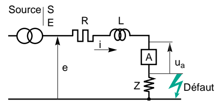
Fig. 2 : schéma de principe d'un circuit en défaut.
