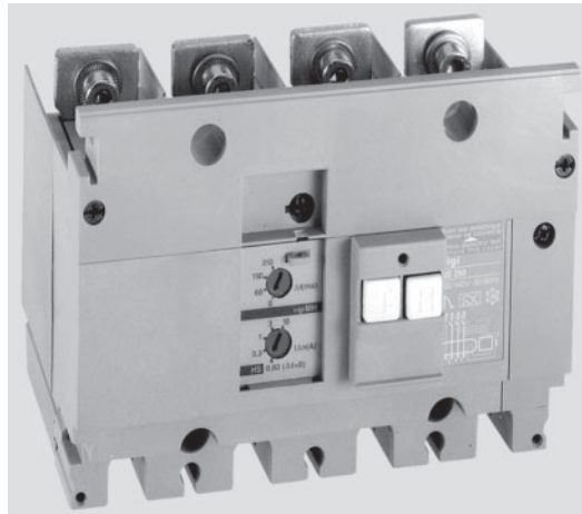
Fig. 23 : Vigi module of a Compact NS.
