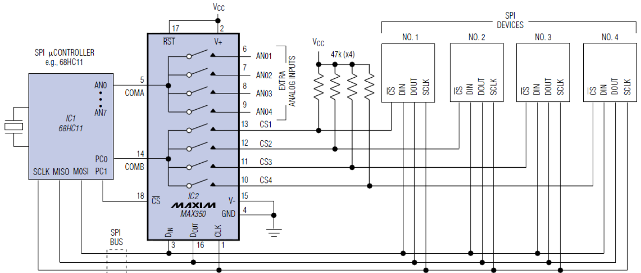
Figure 1. Un multiplexeur double à 4 canaux accroît le nombre de canaux et d'entrées de sélection pouvant être utilisés par ce microcontrôleur.
