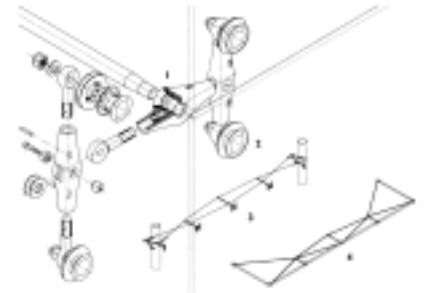
Système d'attache des verres d'un mur-rideau suspendu. Serres de la Cité des sciences et de l'industrie à Paris, Adrien Fainsilber, Peter Rice.
