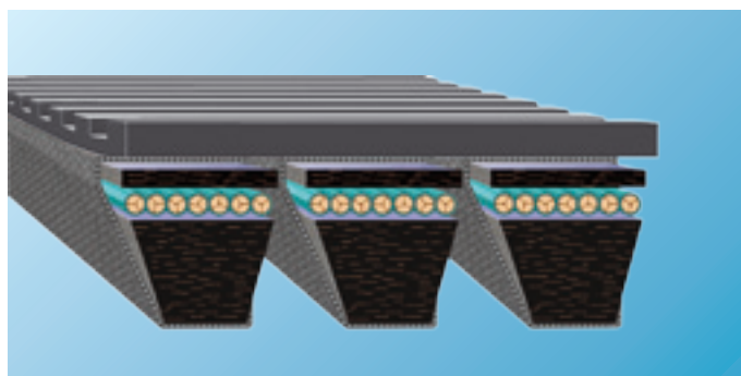
Courroie jumelée avec revêtement PKR 1
