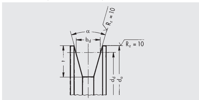
Poulie de mesure pour courroies trapézoïdales étroites de haute capacité DIN 7753 Partie 1 et courroies trapézoïdales classiques DIN 2215
