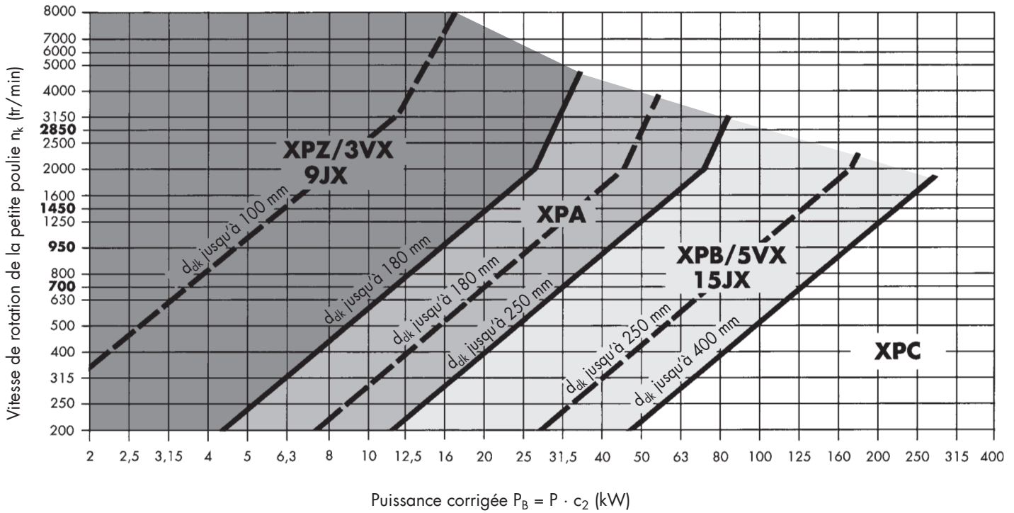
Diagramme 4: Courroies trapézoïdales étroites Optibelt Super X-POWER M=S
