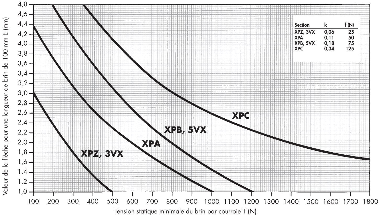
Diagramme 10: courbes de tension initiale des courroies trapézoïdales étroites Optibelt SUPER X-POWER M=S – flancs nus, crantées moulées
