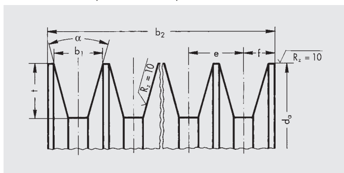
Poulie de mesure pour courroies jumelées
