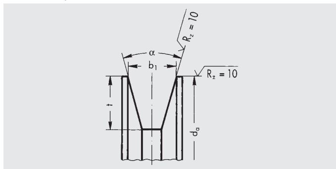
Poulie de mesure pour courroies trapézoïdales étroites de haute capacité norme américaine RMA/MPTA
