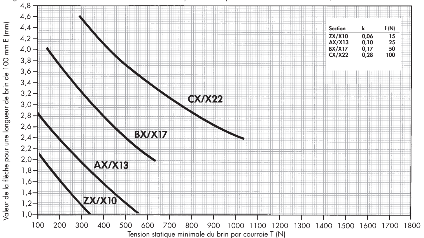
Diagramme 11: courbes de tension initiale des courroies trapézoïdales Optibelt SUPER TX M=S – flancs nus, crantées moulées
