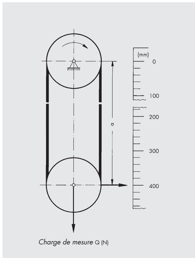
Poulie de mesure pour courroies jumelées
