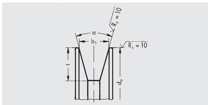
Poulie de mesure pour courroies hexagonales
