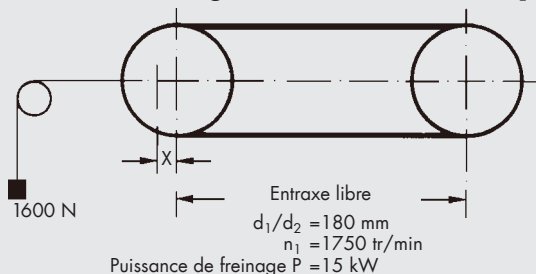
Banc d'essai - augmentation de l'entraxe [mm]
