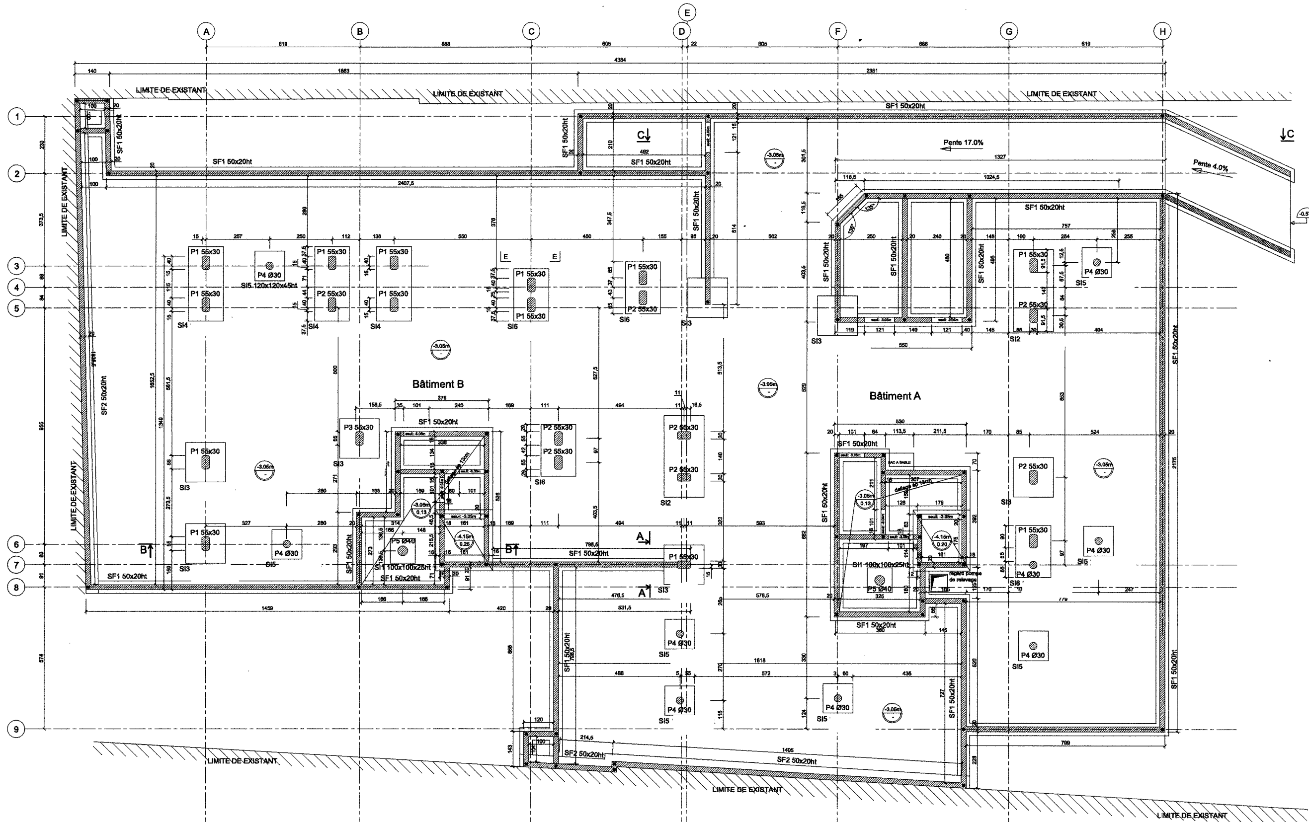
DB6 PLAN DE FONDATIONS Echelle: 1/150
