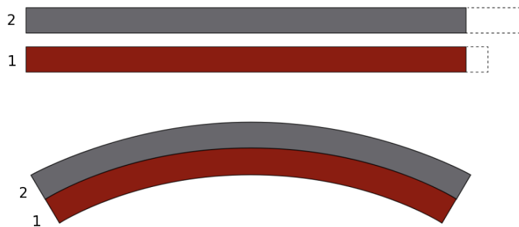
Figure 13 : Constitution d'un bilame et déformation sous l'effet de la chaleur, source [10]
