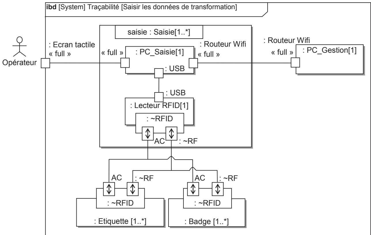
Figure n°5 : diagramme de bloc interne partiel
