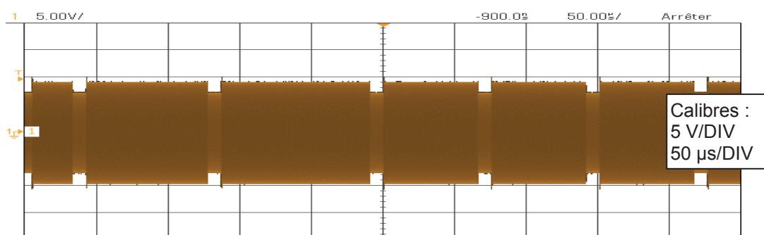
Figure n°8 : relevé d'une transmission vers une étiquette I•CODE SLI (NXP)
