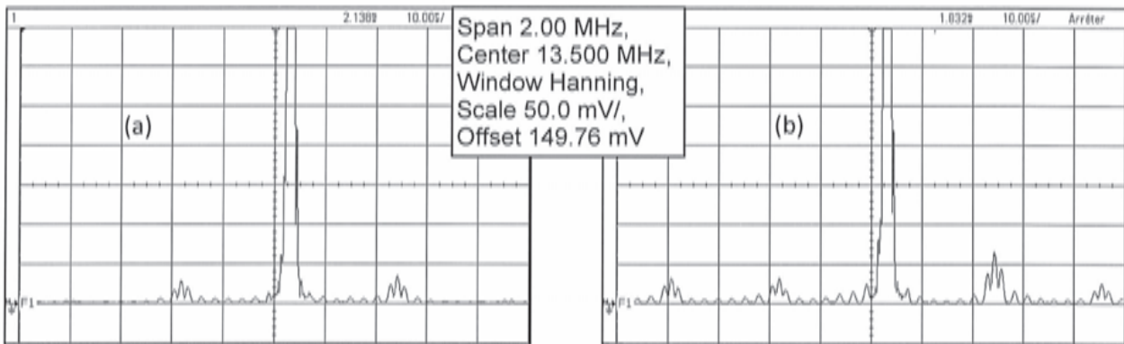
Figure n°15 : spectre relevé pour les deux situations de communication
