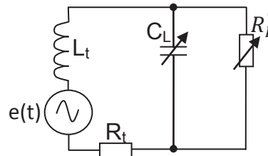
Figure n°24 : modèle équivalent simplifié du TAG seul
