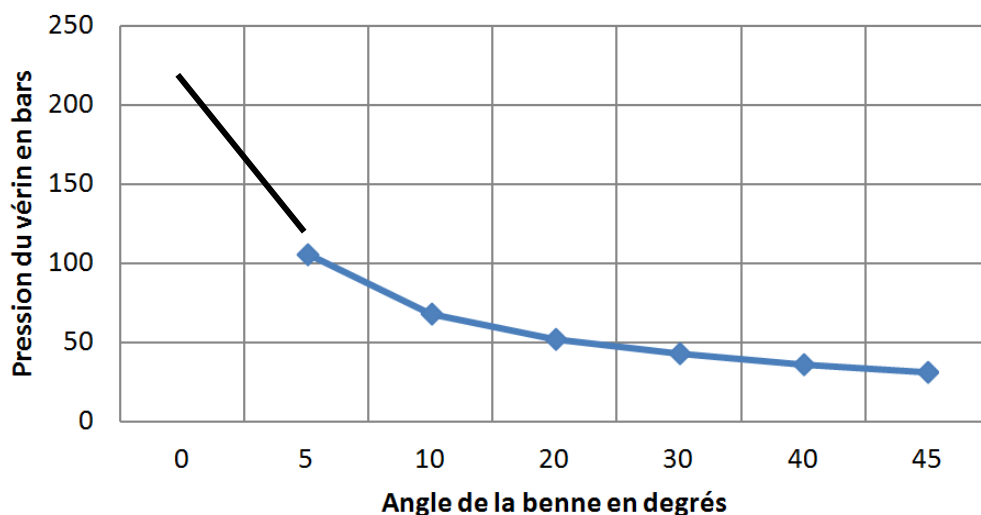
Pression dans le vérin en fonction de l'angle de la benne
