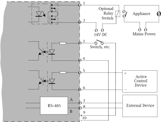
Connecteur E/S 10 broches : exemple d'application.
