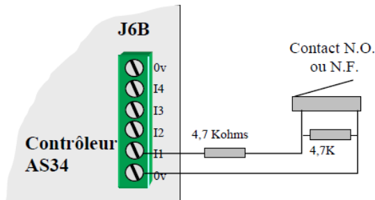
Fig. 5 : Exemple de connexion d'un contact sur l'entrée I1.
