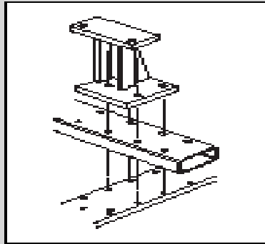
Fig. 4. Elements dissociés
