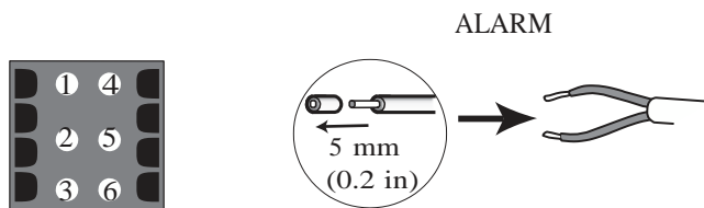
Figure 4.4 Broches des connecteurs d'alarme et de relais
