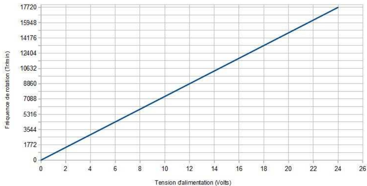
Evolution de la fréquence de rotation en fonction de la tension d'alimentation
