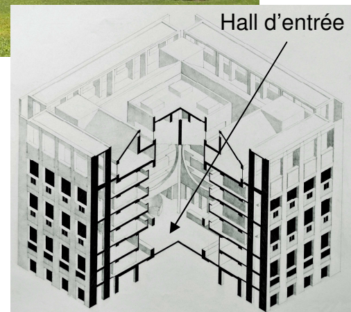
3.2 Vue en perspective axonométrique
