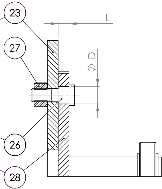
COUPE F-F ECHELLE 1 : 2
