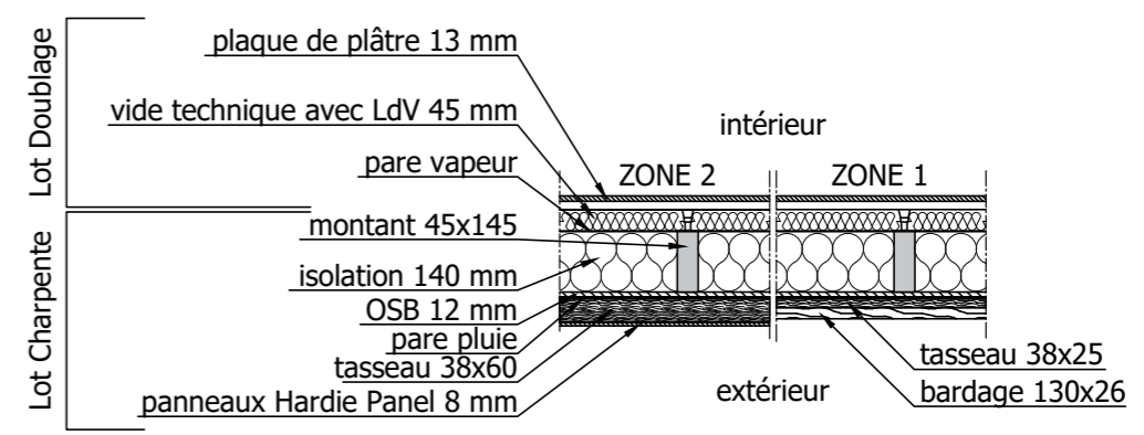
Coupe horizontale sur ossature
