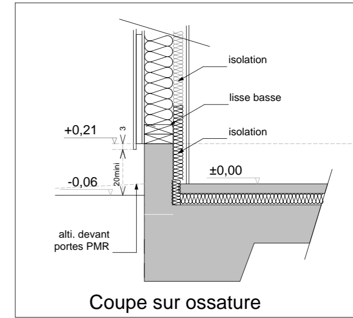
Coupe sur seuil encastré
