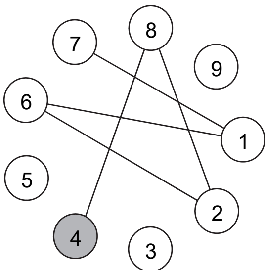
Figure 1. Un chemin de longueur 5 depuis le nombre 4
