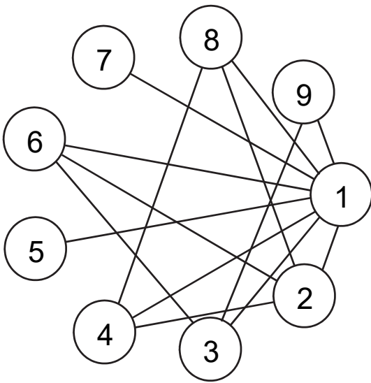
Figure 4. Le graphe du jeu à 9 entiers
