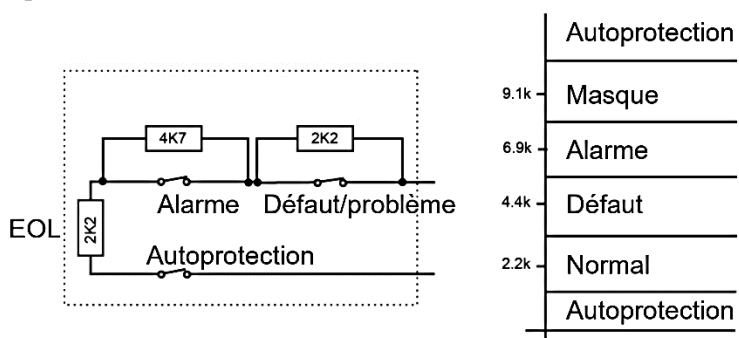
Figure 4. Connexions ZFS avec masquage
