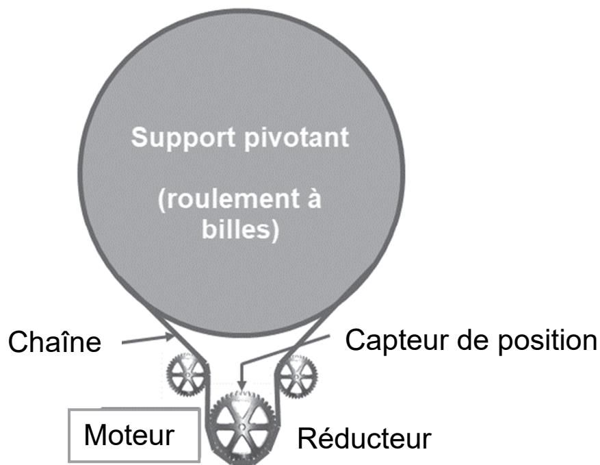
Figure 2 : système de rotation
