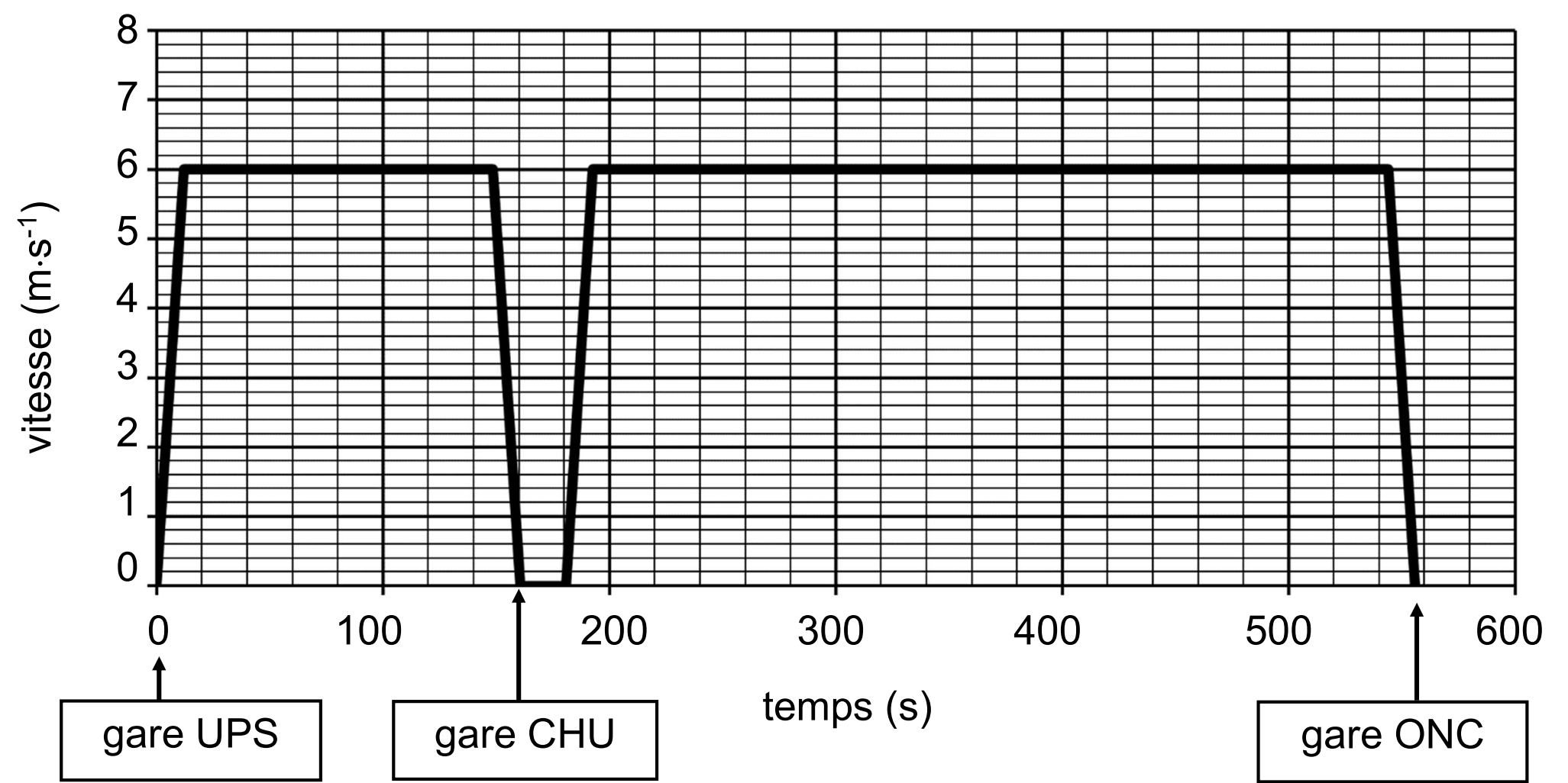
Graphe des vitesses – Vitesse 1
