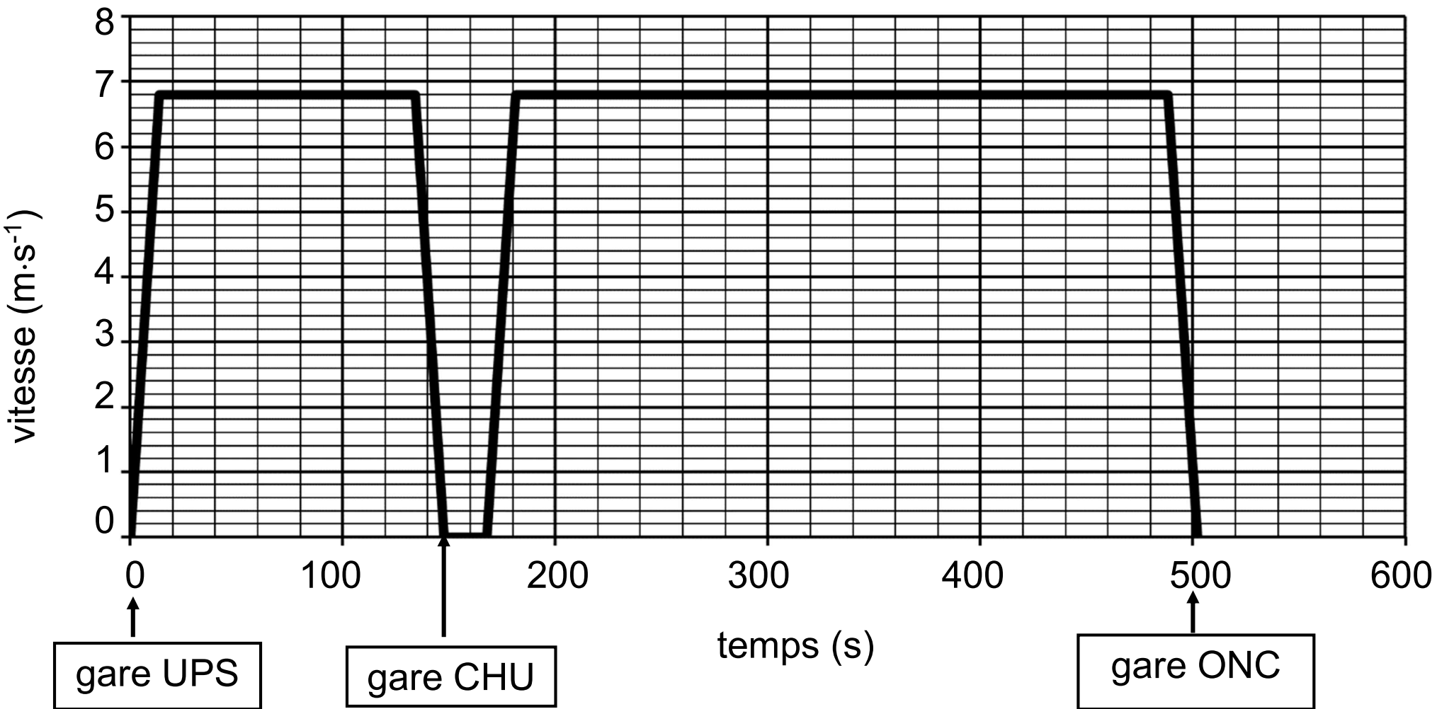
Graphe des vitesses – Vitesse 2
