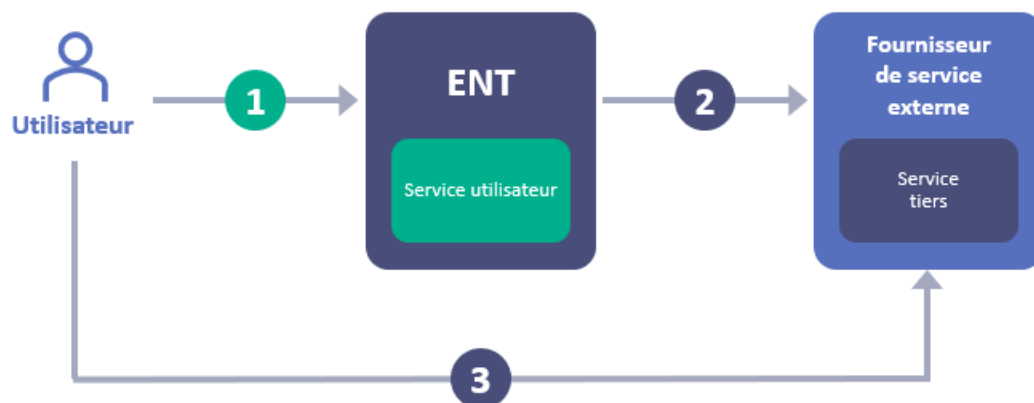
Figure 8 : Cinématique fonctionnelle pour les services de catégorie 1
