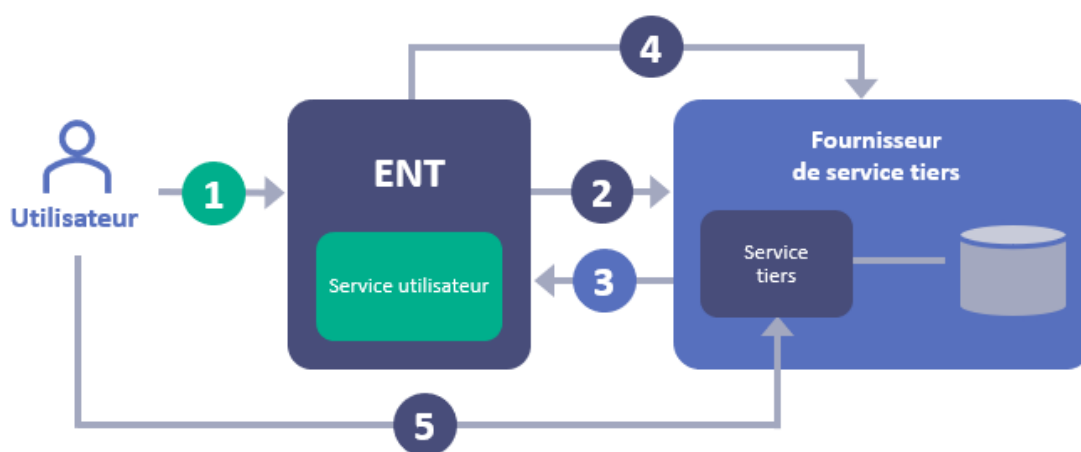
Figure 12 : Cinématique fonctionnelle pour les services de catégorie 4 (cas de la connexion nominale)
