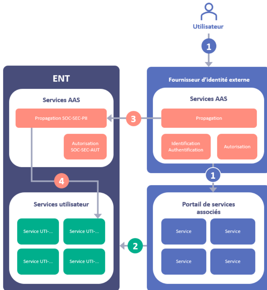
Figure 6 : Authentification déléguée à un fournisseur d'identité externe et accès à un service ENT depuis un portail externe
