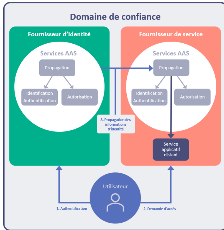
Figure 3 : Propagation des informations d'identité
