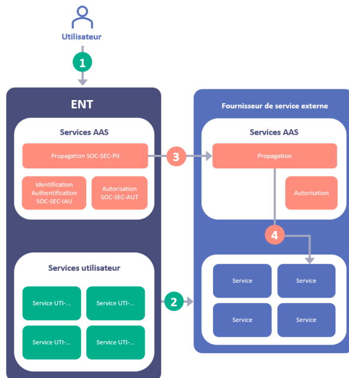
Figure 7 : ENT fournisseur d'identité et accès à un service externe depuis le portail de l'ENT
