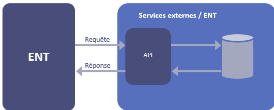
Figure 15 : Echanges entre l'ENT et les services externes de l'ENT via API
