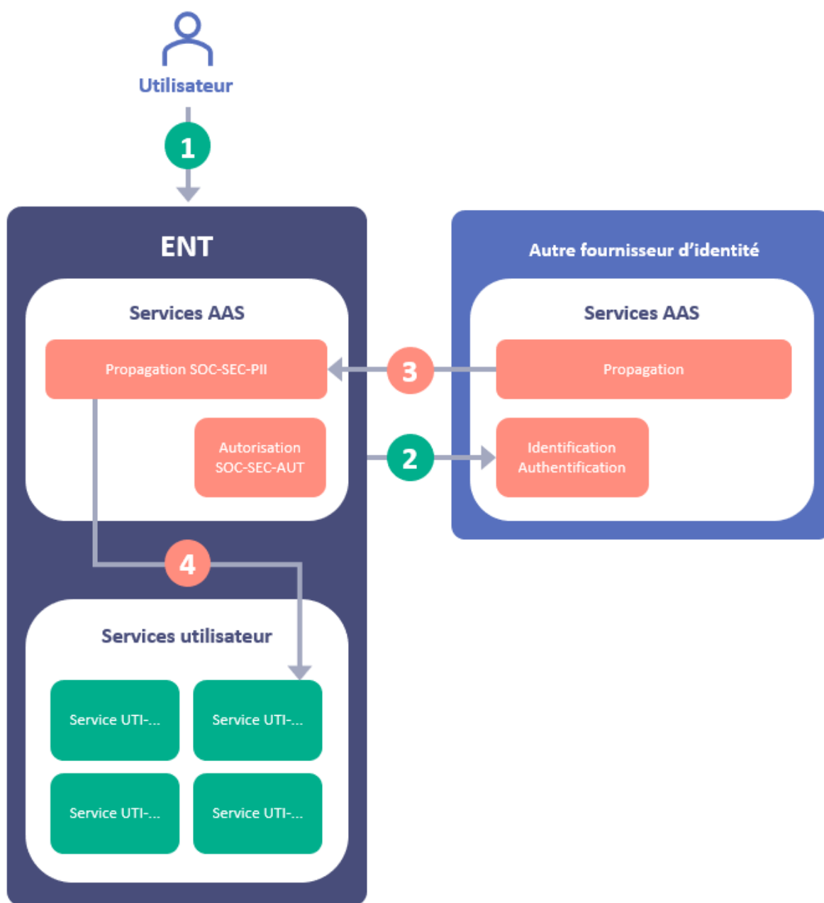
Figure 4 : Authentification déléguée à un fournisseur d'identité externe et accès à un service ENT depuis le portail de l'ENT
