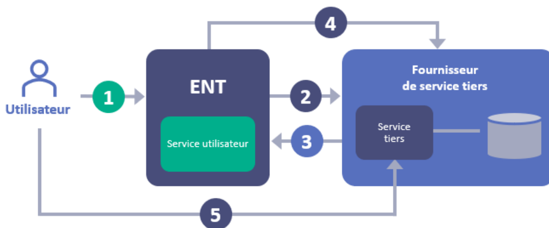
Figure 14 : Cinématique fonctionnelle pour les services de catégorie 5 (cas de la connexion nominale)
