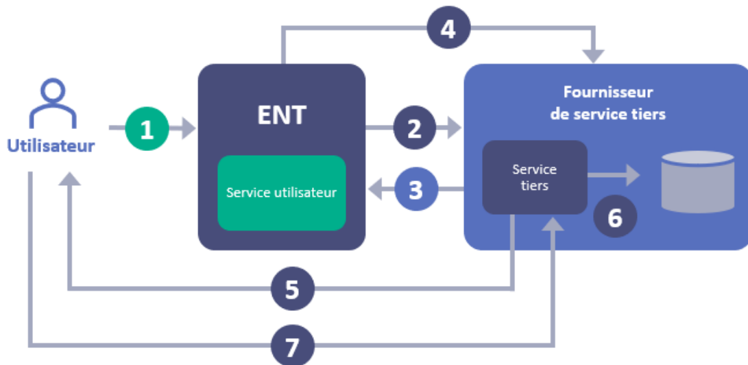
Figure 13 : Cinématique fonctionnelle pour les services de catégorie 5 (cas de la première connexion)
