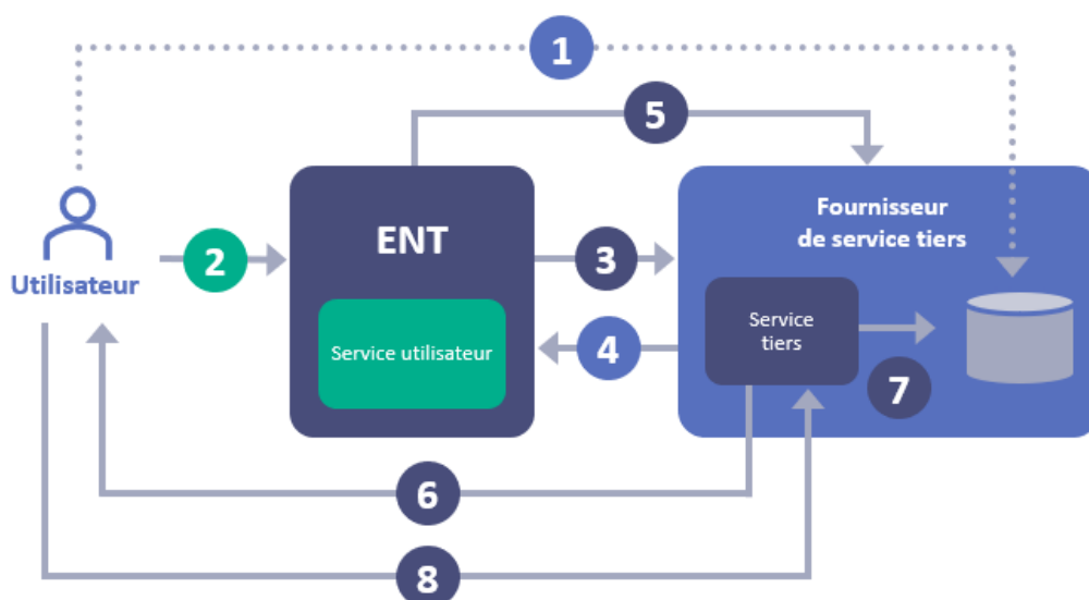
Figure 11 : Cinématique fonctionnelle pour les services de catégorie 4 (cas de la première connexion)
