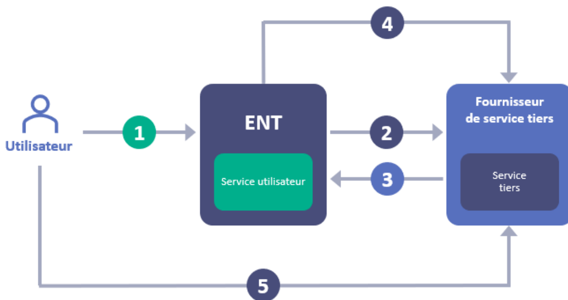
Figure 9 : Cinématique fonctionnelle pour les services de catégorie 2
