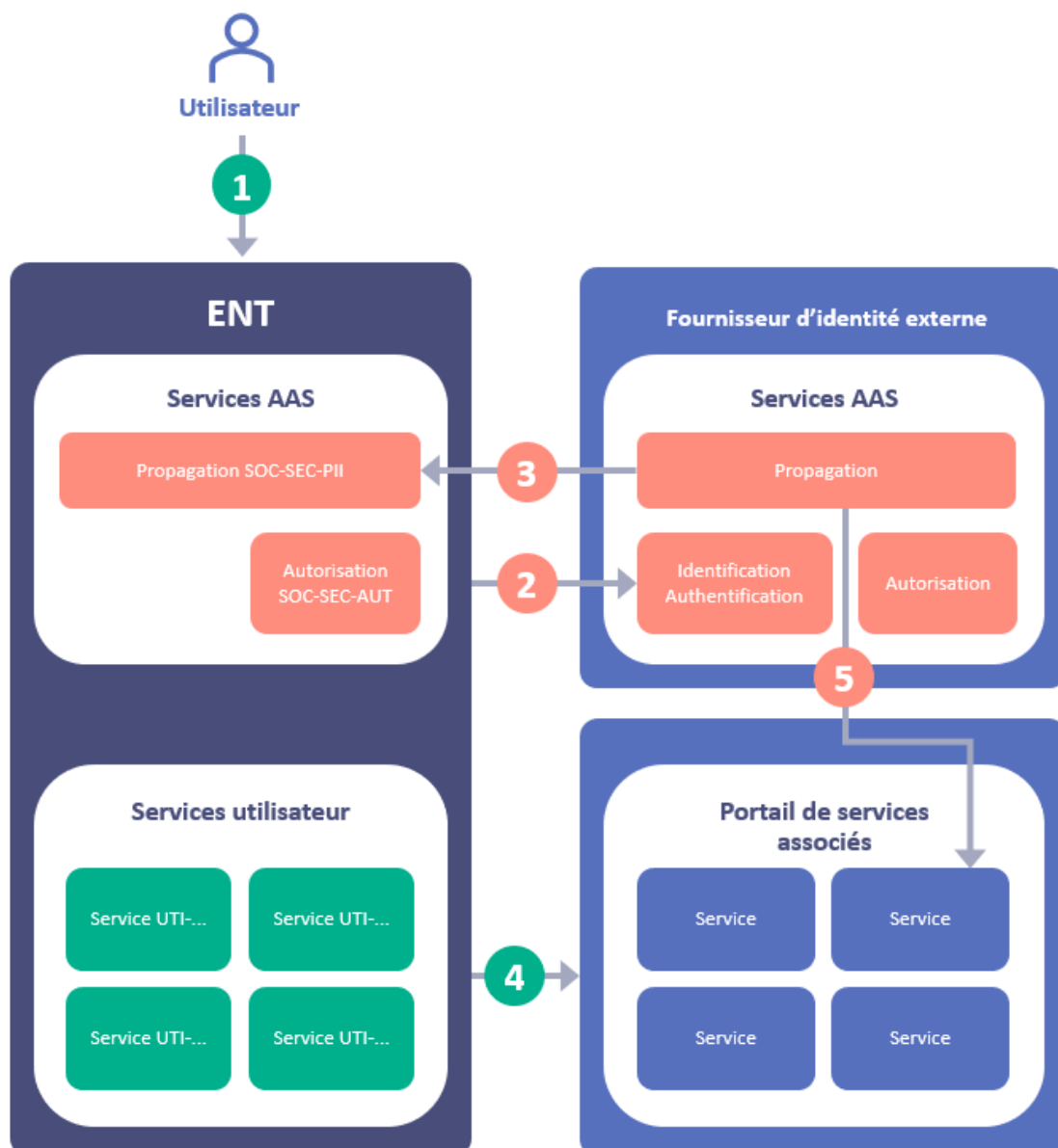
Figure 5 : Authentification déléguée à un fournisseur d'identité externe et accès à un fournisseur de service externe depuis le portail de l'ENT
