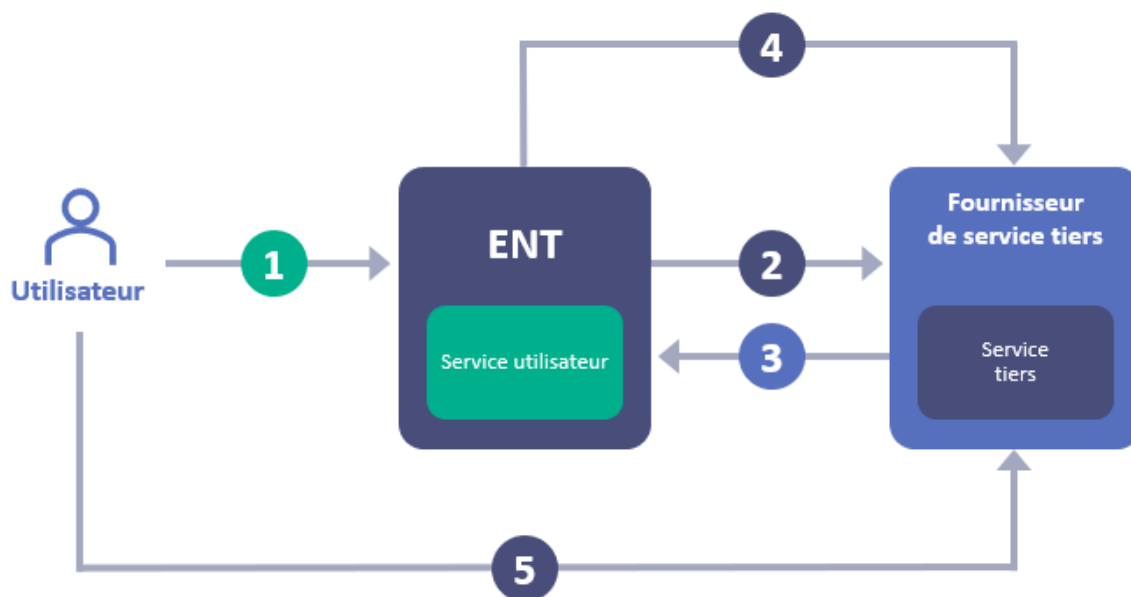
Figure 10 : Cinématique fonctionnelle pour les services de catégorie 3
