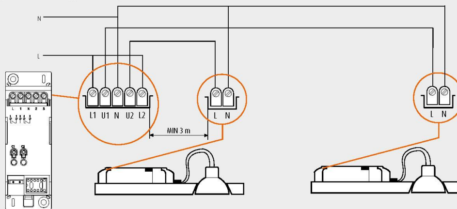
Schéma pour le raccordement d'appareils d'éclairage
