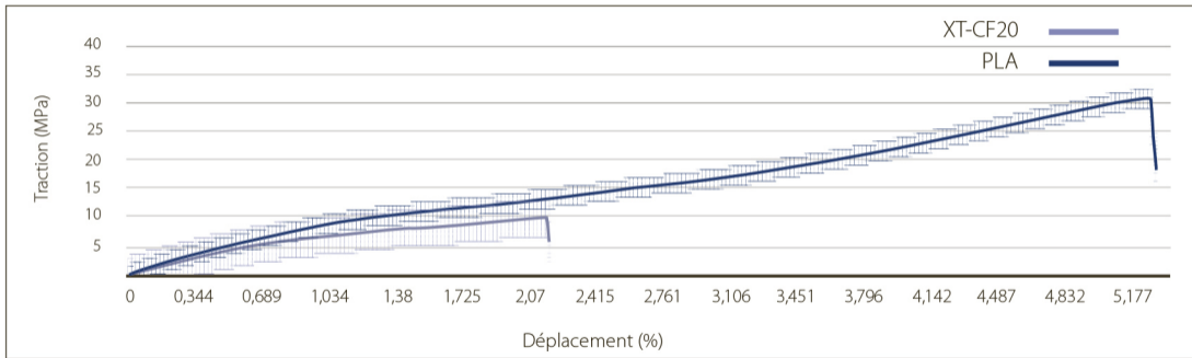
14 Résultats du troisième test de traction (traction 45°)
