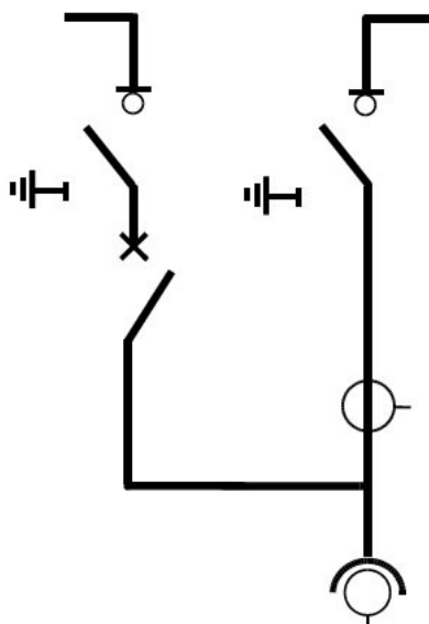
Image 20 Cellule de comptage HTA Catalogue Uniswicht
