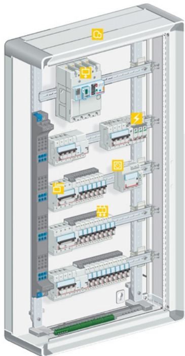
Coffret divisionnaire
