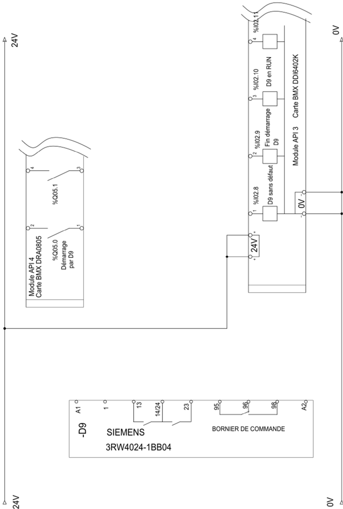
DRA3 : Schéma de commande du démarreur D9 et des entrées sorties API
