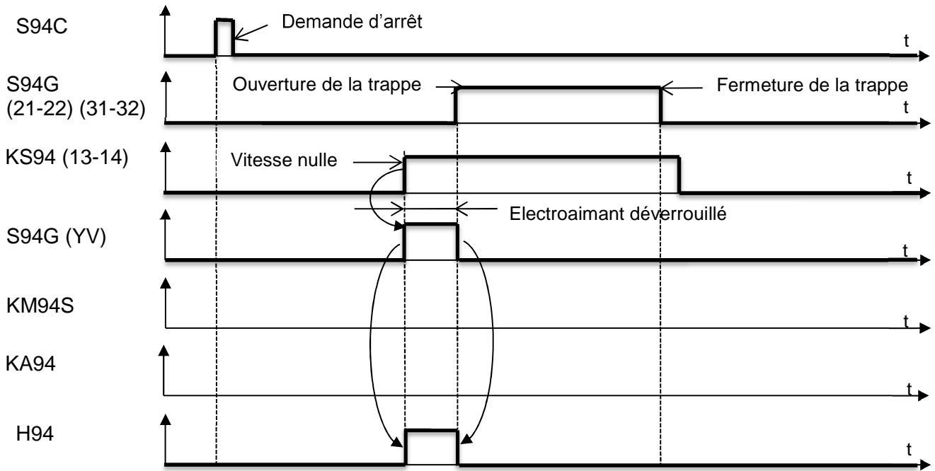
DRC2 : Chronogramme de fonctionnement de la nouvelle solution de sécurité
