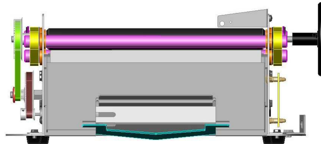
Vue de face avant de la plieuse
